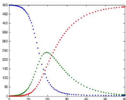
Figura n.º3. Un ejemplo de modelo SIR (Azul = Población susceptible, Verde= Población infectada y Rojo = Población recuperada). Fuente: No machine-readable author provide; Dominio público; File:Sirsys-p9.png.
