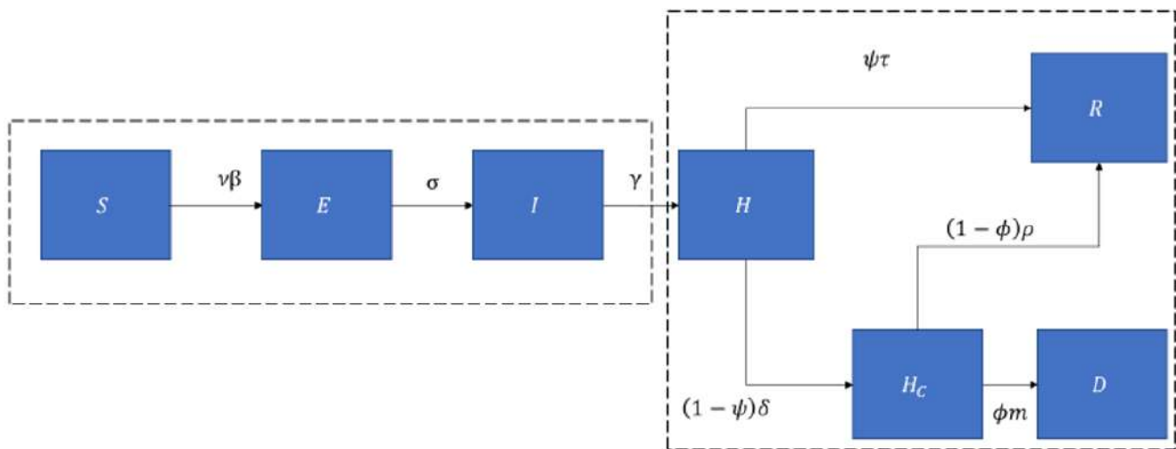
Figura n.º 4. Diagrama del modelo compartimental SEIR modificado
